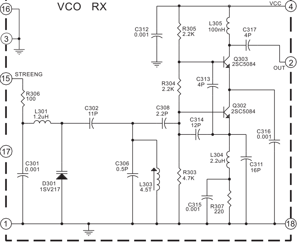
V.C.O. (148-174MHz) 770-030-0017
